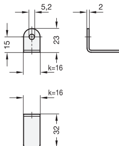
Laschenbreite k=16
