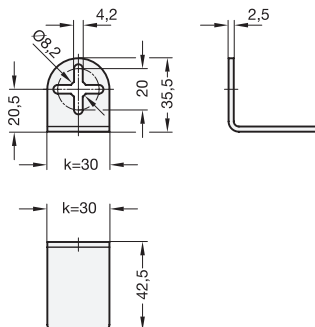
Laschenbreite k=30
